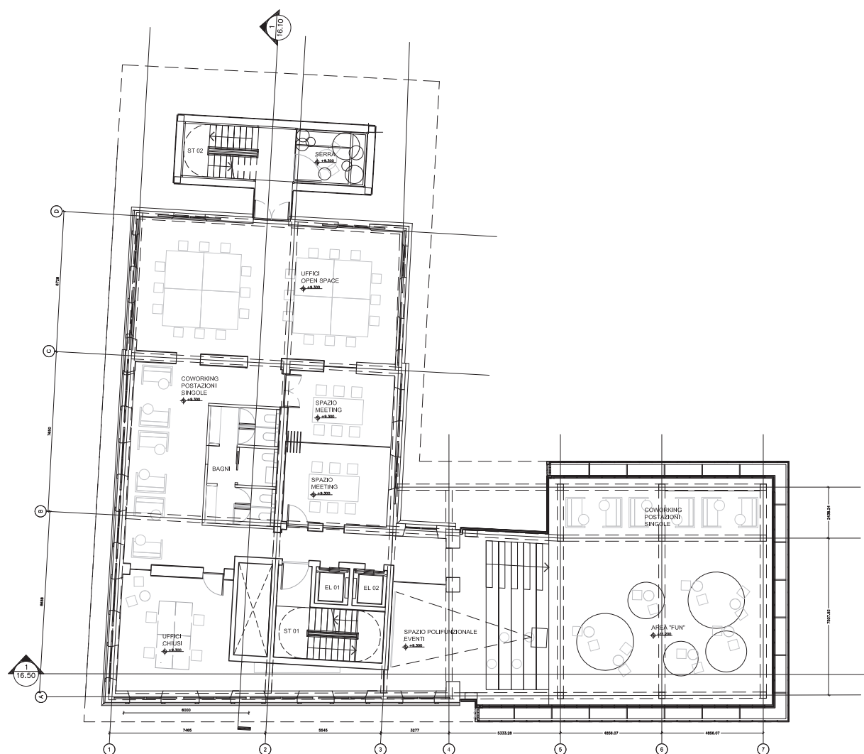
STRUTTURA IN LEGNO
